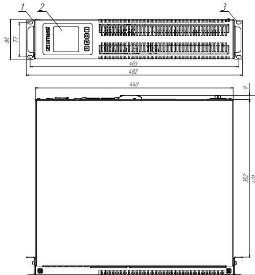
Рисунок 4а. Габаритные размеры и компоненты ИБП Штиль STR1101L, STR1101SL и STR1101LD (горизонтальная установка в стойку)
